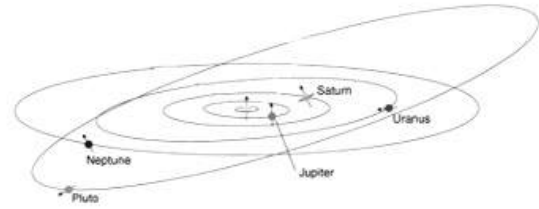
Pluto nunc non iam habetur ut planeta (www.cnes.fr)
