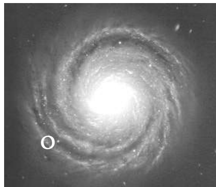
Via lactea (in circulo est Sol).
