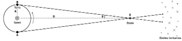
Schema parallaxis annuæ. (in «De immenso cælo IV - Wikipedia)
