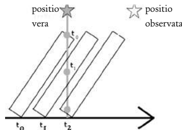
In hoc schemate monstratur tubus telescopii in motu secundum sagittam; in prima positione non recipit lucis radium a stella verticaliter provenientem, sed solum in positione t_2 , quo fit ut stella videatur esse alio loco (astronomie-smartsmur.over-blog.com).
