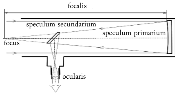
Schema telescopii a Newtono fabricati ( astronomie-amateur.sophie.m.over-blog.com )
