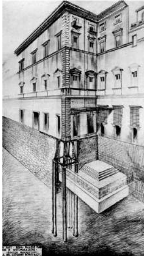
Fulcimentum anguli palatii.
