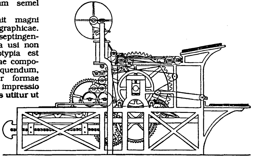
Prelum excogitatum a Koenig, ut thermica agitatum. Fuit inventio maximi momenti, praecipue ad acta diurna imprimenda.
